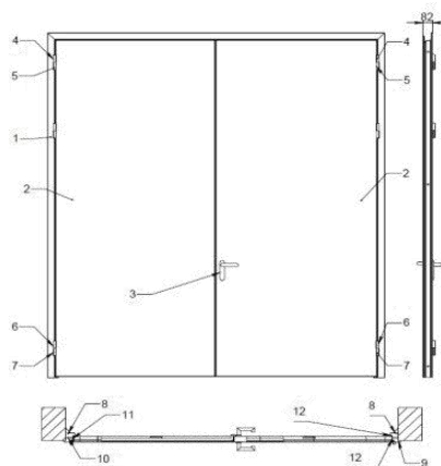
Рис. 1 Ворота противопожарные металлические двупольные
