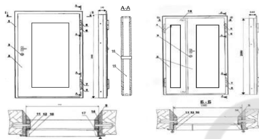
Рис. 1 Двери противопожарные металлические однополюсная и двупольная
